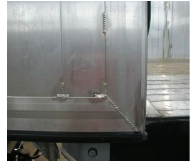
Oldalajtók: hegesztési varratok ellenőrzése, van-e repedés
