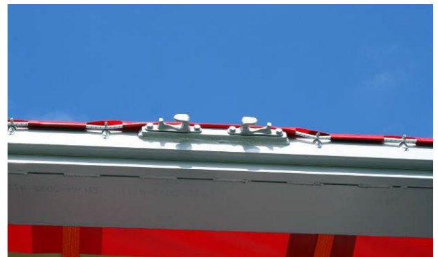
Hátsó ajtó felül: a zárcsapon van-e sérülés, csavarok megfelelő rögzítettsége
