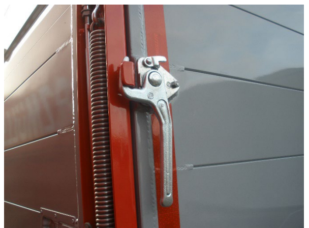
Zámek: zkontrolovat funkčnost a opotřebení.
