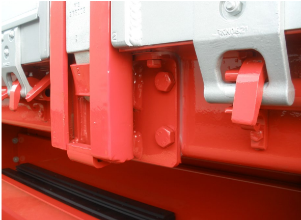
Uložení sloupků: zkontrolovat svary na praskliny a opotřebení pohyblivých dílů. Zkontrolovat upevnění šroubů.
