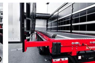
T Kitekerhető portálkeret
