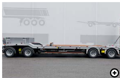
1 Hajlított plató Ennek köszönhetően a mélybölcsős részen a rakodási magasság nagyon alacsony lesz. Ennek eredményeként magasabb járművek is szállíthatók.
