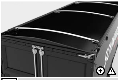
14 Dachbogen Die materialabweisenden und runden Dachbögen bringen zusätzliche Stabilität in die Kippmulde. Diese sind schwenkbar für flexible Beladung und die Neigung reduziert eine mögliche Wassersackbildung.
