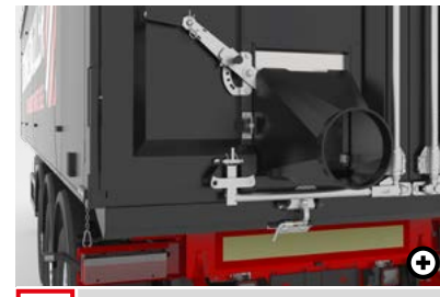
Q Auslaufrichter Der abnehmbare Auslaufrichter in paralleler oder konischer Ausführung für einen gezielten Auslaström.
