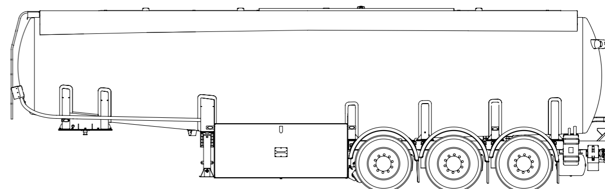
43.500 l Alu-Tankfahrzeug
