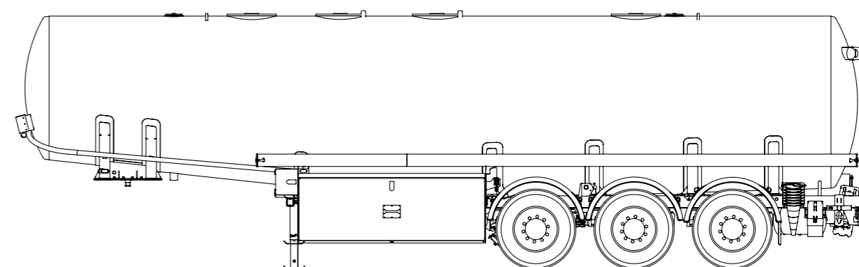
38.000 l Alu-Tankfahrzeug
