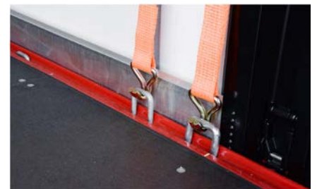
hochschwenkbarer Zurrbügel
